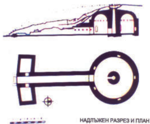
НАДЛЪЖЕН РАЗРЕЗ И ПЛАН
